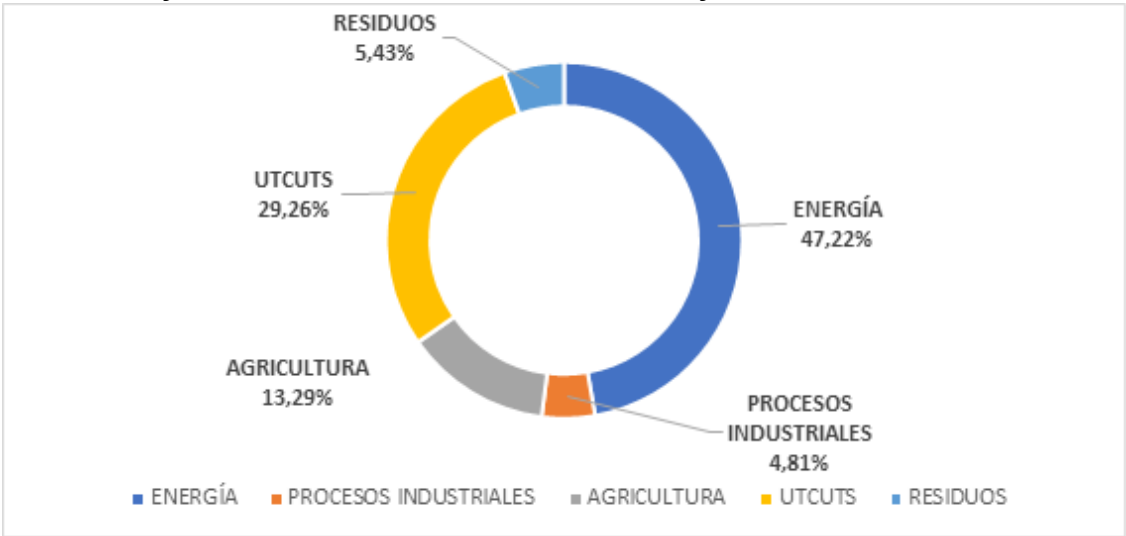
Gráfico 5. Inventario Nacional de Gases de Efecto Invernadero 2022
