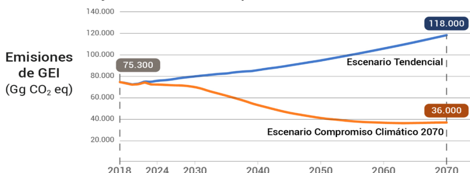
Gráfico 4. Escenario Compromiso Climático 2070
